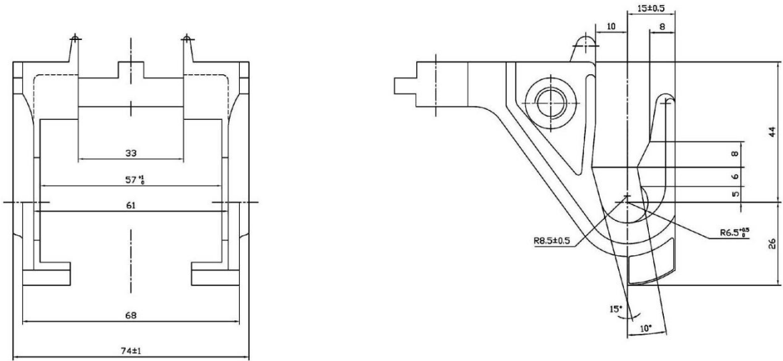
图 A. 4 下触座结构示意图
