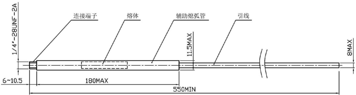
图 A. 5 熔断件（6A-100A）结构示意图
